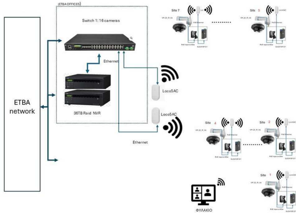
Εικόνα 3: Διάγραμμα σε σημεία με παροχή ρεύματος – Ε.Π. Ξάνθης
